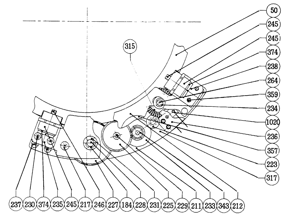
C-C (2:1)
